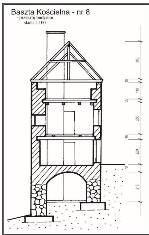
inwentaryzacja baszty kościelnej
